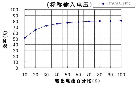
效率VS输出负载曲线图
