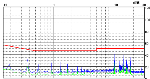
E2415S-1WR2 传导骚扰 Class B 测试效果图 (正线)
