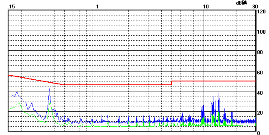
F2405S-1WR2 传导骚扰 Class B 测试效果图 (负线)
