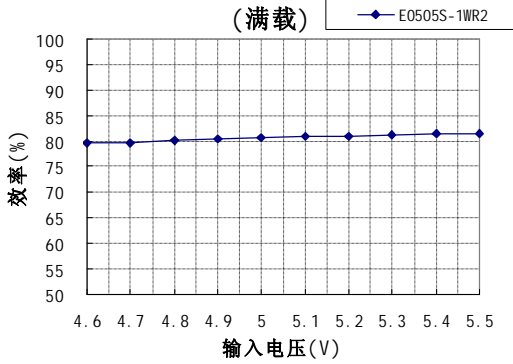
效率VS输入电压曲线图
