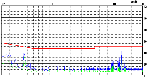
F2405S-1WR2 传导骚扰 Class B 测试效果图 (正线)
