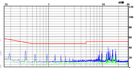
E2415S-1WR2 传导骚扰 Class B 测试效果图 (负线)
