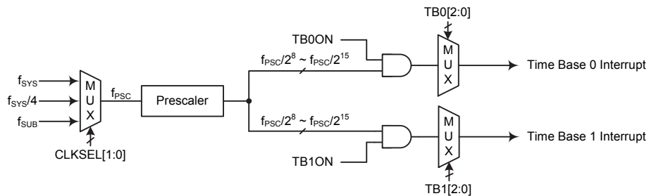
时基中断
