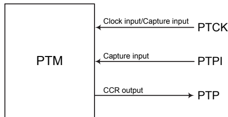
PTM 功能引脚控制方框图
