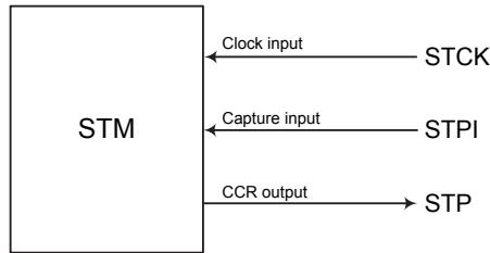
STM 功能引脚控制方框图
