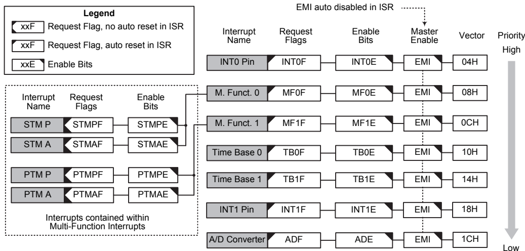
中断结构
