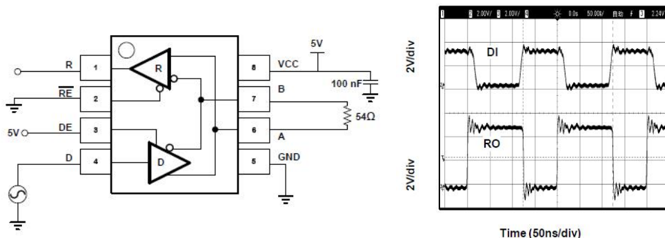
图15 回环测试及其波形
