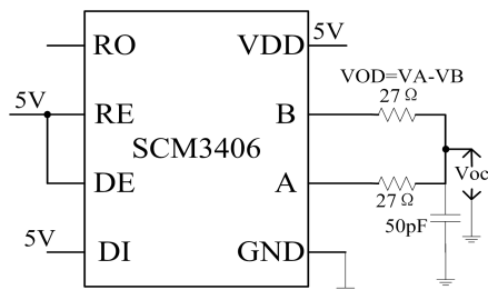
图 18 驱动器 V_{oc} 输出测试电路及波形
