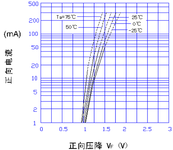
附图2. 正向电流与正向压降关系
