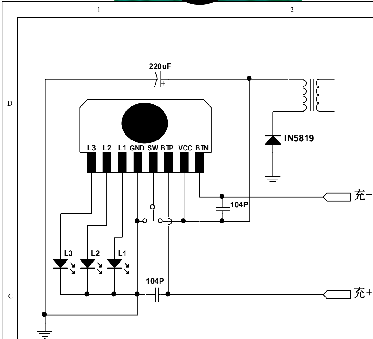
图 3 TC3582DA 三灯、七彩模式任选
