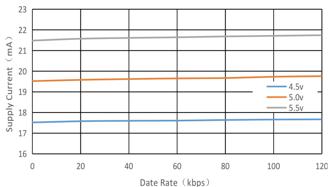
图4. 工作电流与通讯速率的关系
