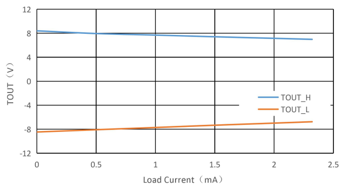
图2. 发送器输出高/低电平与负载电流的关系
