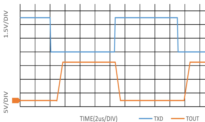
图6. 120kbps 的数据传输 ( V_{CC}=3.3V , R_L=3k\Omega )
