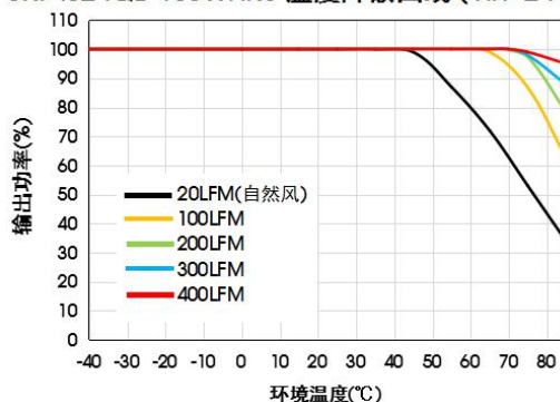
URF4824QB-150WHR3 温度降额曲线 ( V_{in}=24V )
