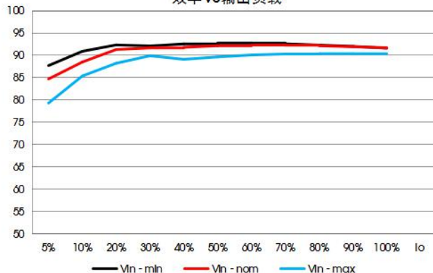
VCF4824EBO-150W(F)R3-N 效率VS输出负载
