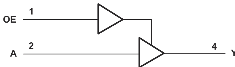
图 9-1. Logic Diagram
